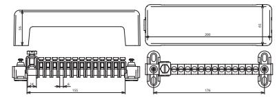
Maßbild PAS AH RK 13X25 1X8.10
