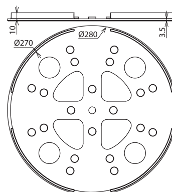
Maßbild ULP KS D280 SW
