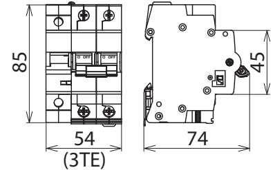
Maßbild POP 2 255 C40
