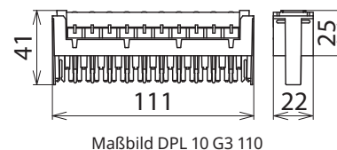
Maßbild DPL 10 G3 110
