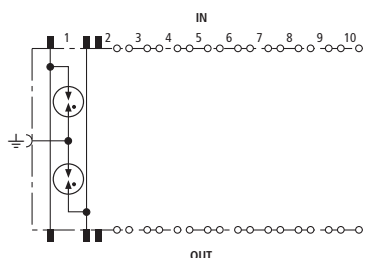
Prinzipschaltbild DPL 10 G3 110
