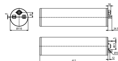
Maßbild DASD 45 LP 100 T
