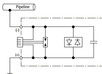
Prinzipschaltbild DASD 45 LP 100 T
