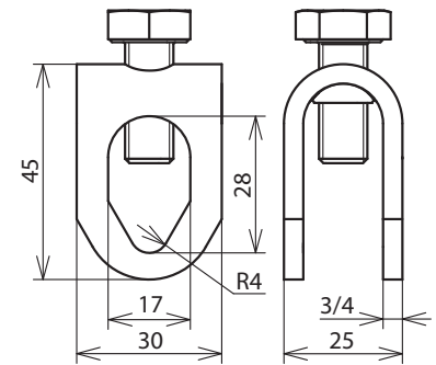
Maßbild FSK 8.10 16 SKM10X25 V2A
