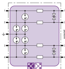
Prinzipschaltbild BXT ML4 BD EX 24
