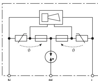
Prinzipschaltbild STC 230
