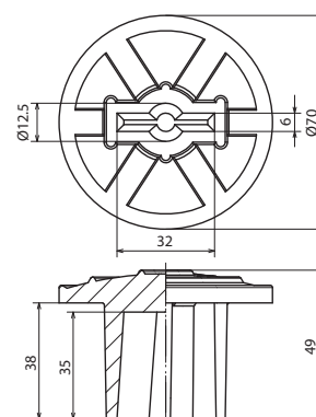
Maßbild SK RD10 FL30X3.5 GRGE PVC
