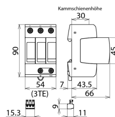
Maßbild DG M WE 600 FM
