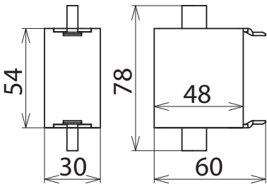
Maßbild DBM NH00 255
