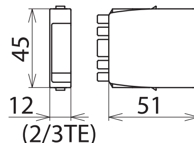
Maßbild BXT ML2 B 180
