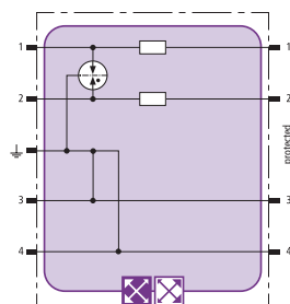
Prinzipschaltbild BXT ML2 B 180
