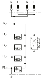
Prinzipschaltbild DSH ZP 2 LSG A TT 255
