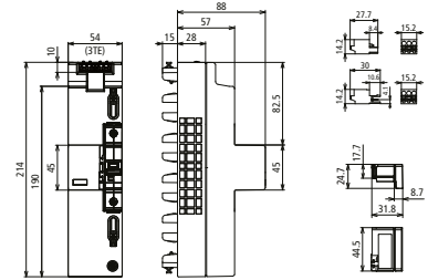
Maßbild DSH ZP 2 LSG A TT 255
