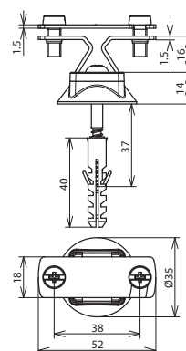
Maßbild FBH ZS 30 KS KD8X40 V2A
