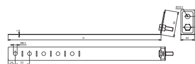
Maßbild RRS V 60.150 B10.5 AL
