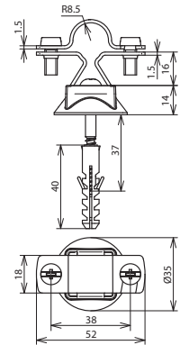
Maßbild SH ZS 16 KS KD8X40 V2A
