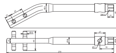
Maßbild RE GK 8.10 SW13 STBRUE
