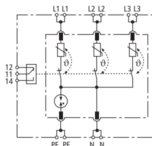
Prinzipschaltbild DR M 4P 255 FM
