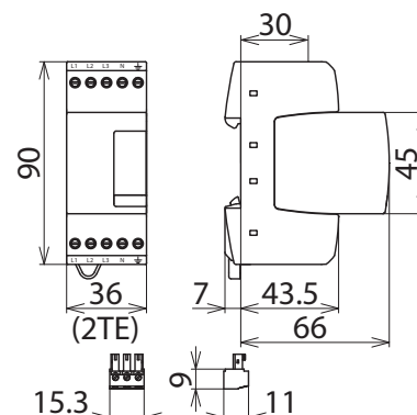
Maßbild DR M 4P 255 FM
