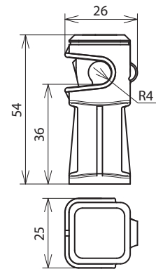
Maßbild LH DS 8 H36 IGM8 GR
