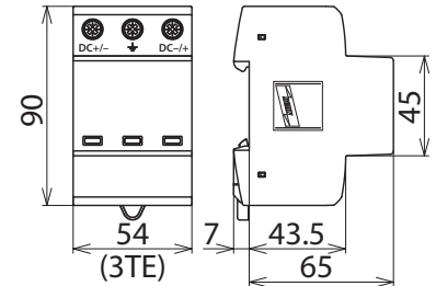
Maßbild
