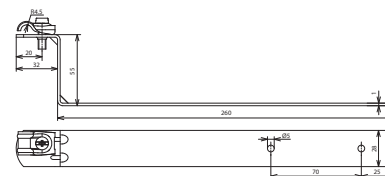
Maßbild DLH DQ 6.10 H55 L260 V2A
