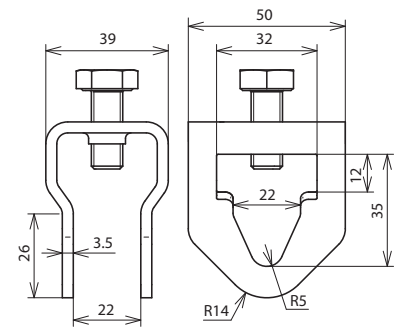
Maßbild AK ES TE 20 RD10 FL30 V4A
