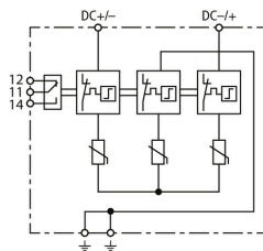
Prinzipialschaltbild DCB YPV 1500 FM
