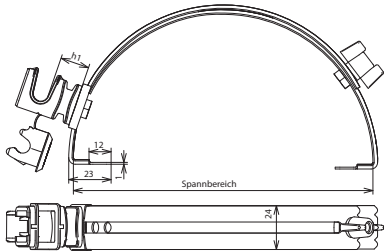
Maßbild DLH DS 8 H36 FG180.280 GR V2A
