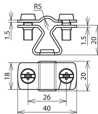
Maßbild LH ZS 8.10 FL20 M8 V2A
