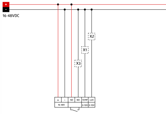
Schaltbild
