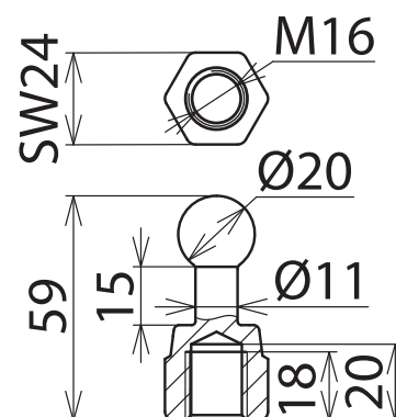
Maßbild KFP 20 M16
