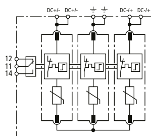
Prinzipschaltbild DCU 2 YPV 1100 3M 1S
