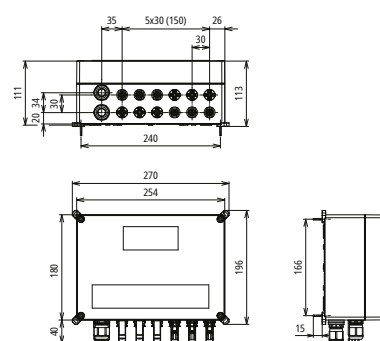
Maßbild DCU 2 YPV 1100 3M 1S MC4 FM
