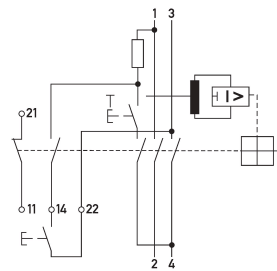
Anschlusschema
