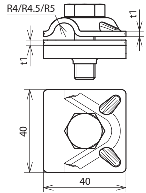
Maßbild
