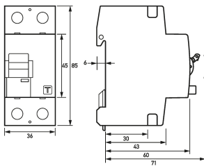
Maßzeichnung Gruppenansicht
