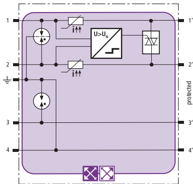
Prinzipschaltbild BXTU ML2 BD S 0-180
