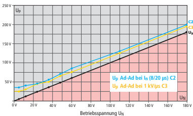
Maßbild BXTU ML2 BD S 0-180
