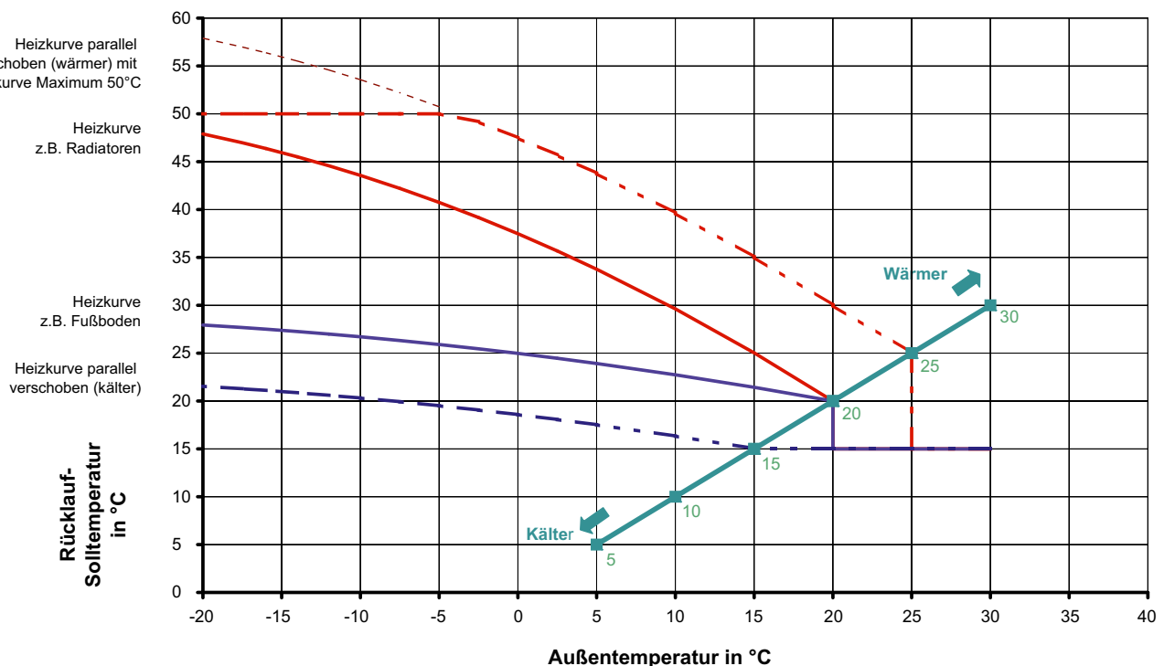
Abb. 3.1: Einstellmöglichkeiten für die Heizkurve
