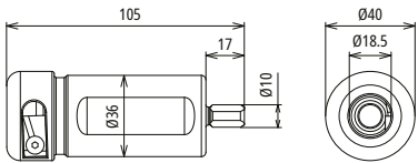
Maßbild ISO HEAD 21
