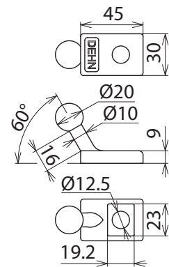
Maßbild KFP 20 S AL 12
