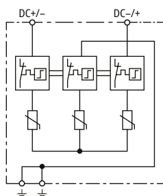
Prinzipschaltbild DCU 2 YPV 1+2 1200 1M
