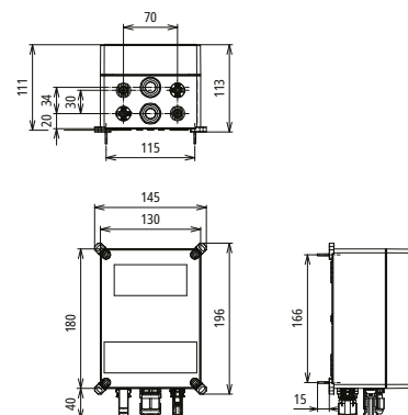
Maßbild DCU 2 YPV 1+2 1200 1M 1S MC4
