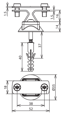
Maßbild
