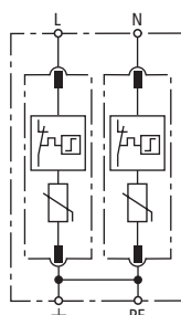
Prinzipschaltbild DG M TN 275
