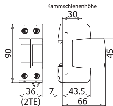
Maßbild DG M TN 275
