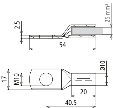
Maßbild PKS 25 10 CUGALNISN
