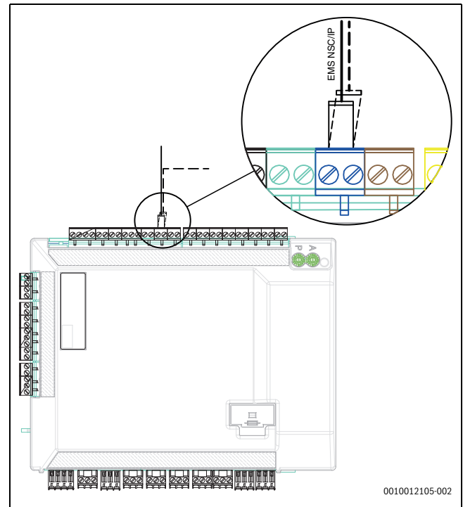
Bild 24 EMS-Anschluss am Installationsmodul
