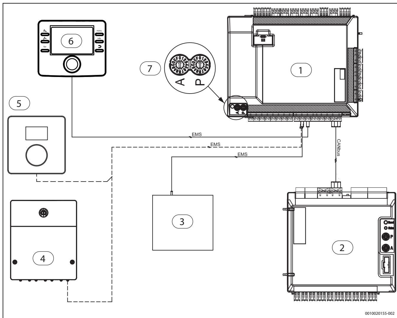
Bild 33 CAN-BUS und EMS – Überblick
