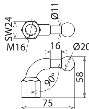
Maßbild KFP 20 W90 M16
