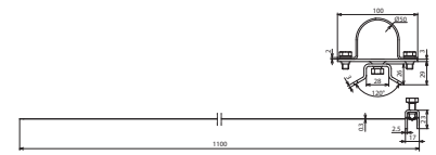
Maßbild BS D50 SB50.300 V2A
